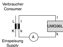
Abb. Anschlussbeispiel: UMG96L mit Ampere-meter in Reihe.
